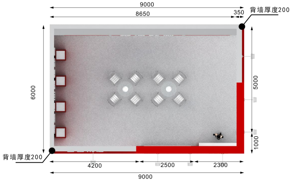
平面图 (单位:mm)
